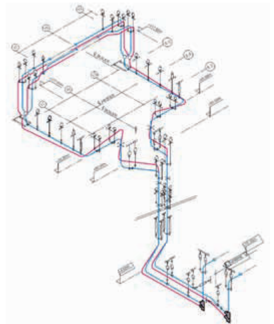
Холодное/горячее положение трубопровода
