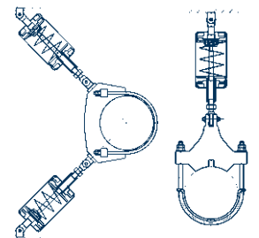
Угловое расположение пружинного блока двустороннего действия типа 27
