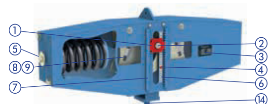
Подвеска постоянного усилия компактной конструкции типа 18
