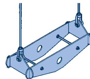
Вертикальный трубный хомут типа 48 с соединениями
