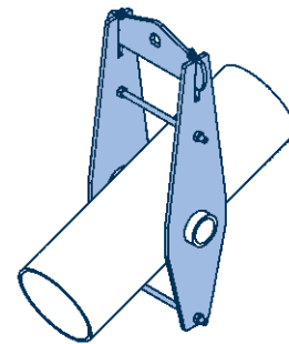
Специальная конструкция типа 48 для трубопровода с наклонным расположением
