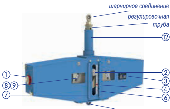
Шарнирная опора постоянного усилия типа 19
