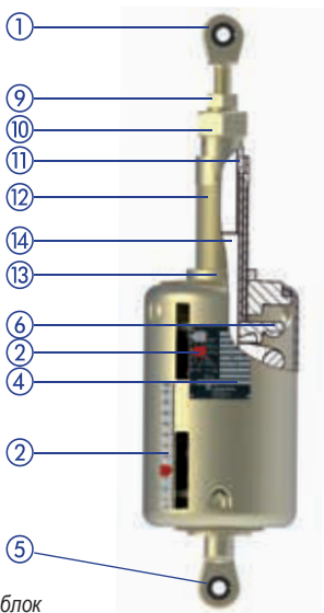
Пружинный блок двустороннего действия типа 27
