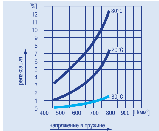
Релаксационные свойства спиральных пружин
