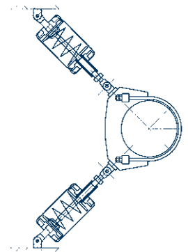
Угловое расположение пружинного блока двухстороннего действия типа 27
