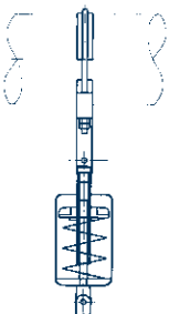
Шарнирная пружинная опора тип 20
