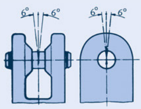
load angle \le 6^\circ
