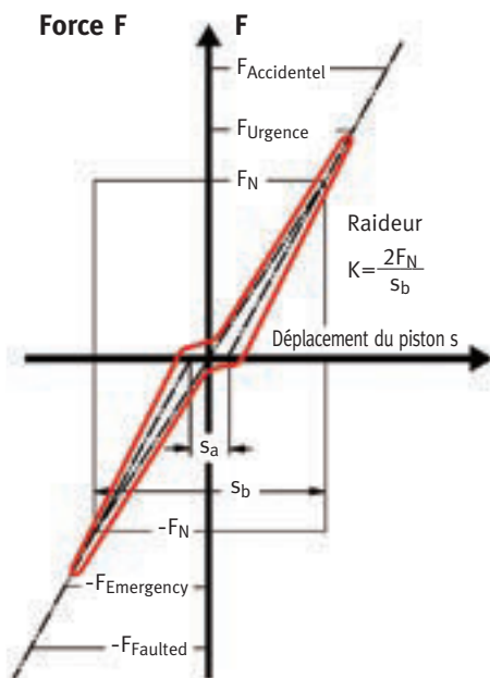
Diagramme Force-déplacement
