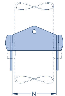
Cote intérieure du caisson (cote-N) du collier vertical Type 46/48
