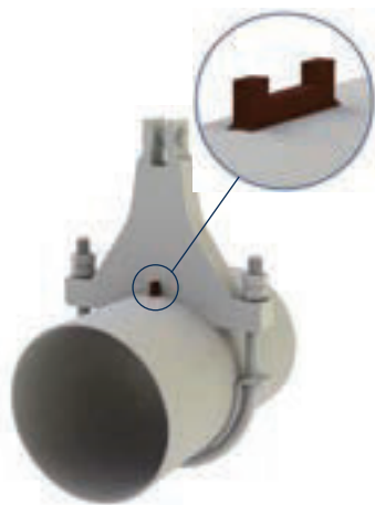
Collier Type 36 avec taquet antirotation Type 3L
