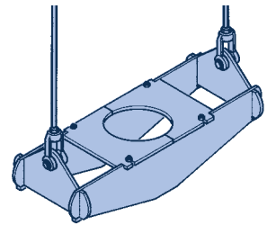
Collier vertical Type 46 avec éléments de raccordement
