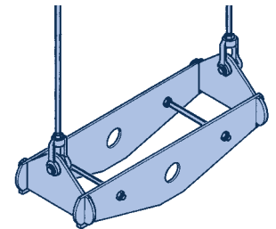
Collier vertical Type 48 avec éléments de raccordement
