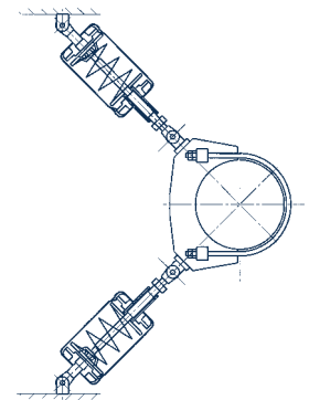
Supports à double effet Type 27 installation en «V»
