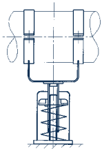
Support variable à charge posée Type 29
