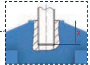
Engagement minimal du filetage «X» du raccordement supérieur (voir tableau de sélection du Type 11, page 1.15)
