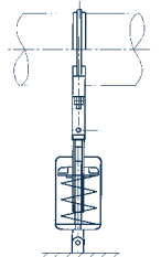
Support à rotules Type 20
