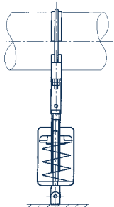
Support variable à rotules Type 20
