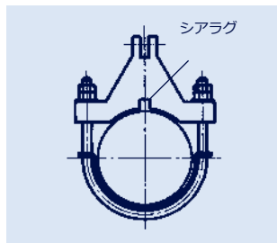
形状接触のクランプ（動的荷重用）
