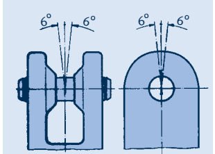
load angle \le 6^\circ
