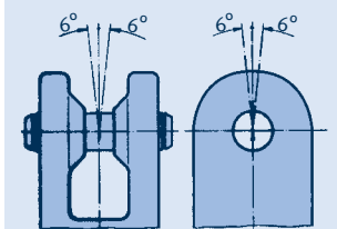
load angle \le 6^\circ
