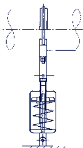
Шарнирная пружинная опора тип 20
