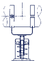
Пружинная опора, тип 29
