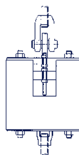
Пружинная подвеска типа 22 с резьбовой серьгой типа 61
