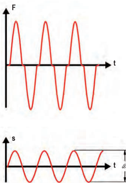
Амплитуды усилия и перемещения
