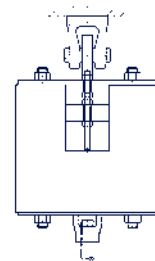
Пружинная подвеска типа 22 с приварной серьгой типа 73
