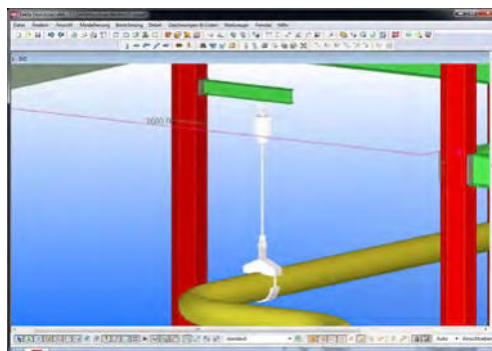
Интерактивно построенная опора в TEKLA Structures
