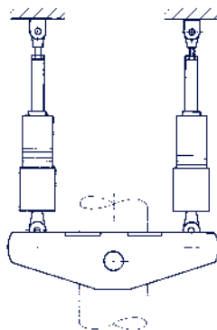
Динамический трубный хомут типа 34 с ударными стопорами и ограничителями поворота.
