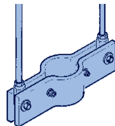
Вертикальный трубный хомут типа 45 с соединениями
