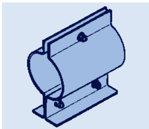
Хомутовые опоры для диаметров труб меньшего размера, типы 49 ... 1, 49 ... 2 до Dy150
