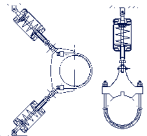
Угловое расположение пружинного блока двухсто- роннего действия типа 27
