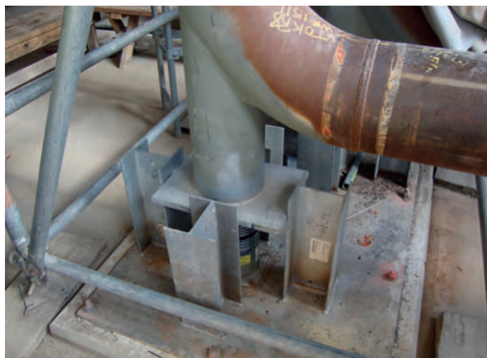
Стойка для колен типа 58 в качестве неподвижной опоры, свободной от моментов относительно осей X-Y с пружинной опорой типа 29
