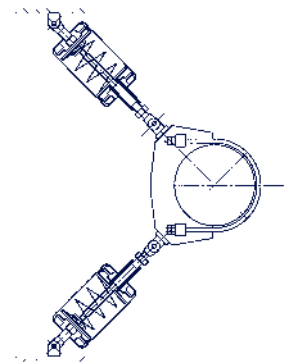
Угловое расположение пружинного блока двухстороннего действия типа 27
