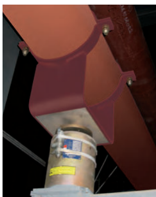
Пластина из нержавеющей стали на основании хомутовой опоры типа 49, теплоустойчивая скользящая подложка и пружинная опора типа 29
