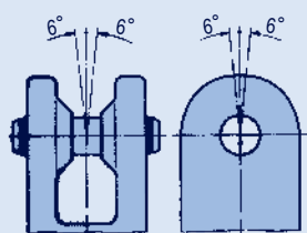
угол нагружения ≤ 6°
