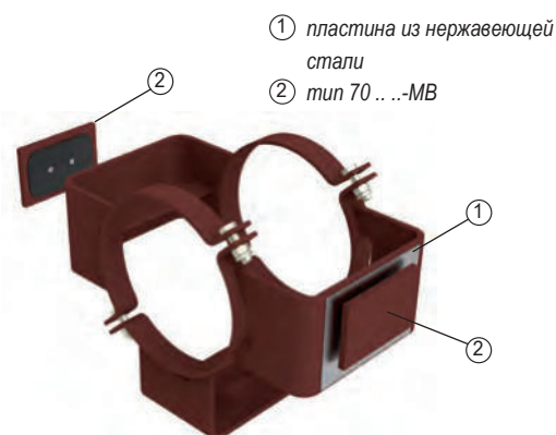
основание/направляющая хомутовой опоры типа 49 ... G3-SP со скользящими подложками
