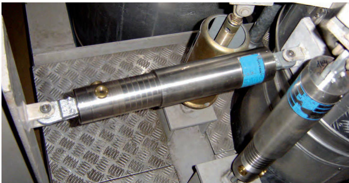
Использование ударных стопоров типа 30
