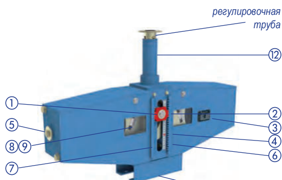
Подвеска постоянного усилия типа 19
