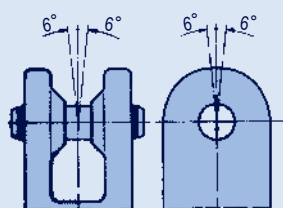
угол нагружения ≤ 6°
