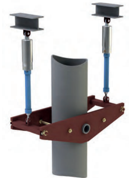
Защита вертикального участка трубопровода с помощью ударных стопоров типа 30 с монтажными удлинителями типа 33 и динамическим трубным хомутом типа 34
