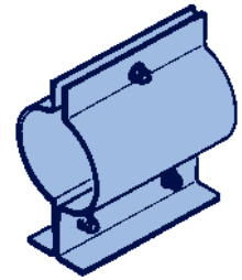
Исполнение 1: Хомутовая опора для низких температур трубы, типы 49 ... 1, 49 ... 2 до Ду 150.
