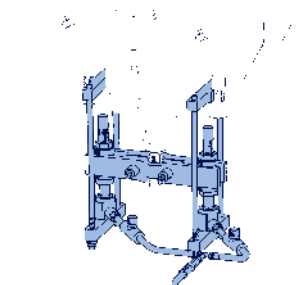
Монтажное устройство, используемое для снятия нагрузки с регулировочной гайки
