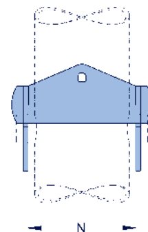
Внутренняя ширина коробки (размер N) вертикальных трубных хомутов типов 46/48
