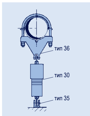
Стандартный случай установки для типа 30
