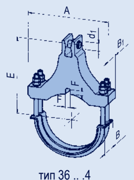
Дн 219.1 (Dy 200)
