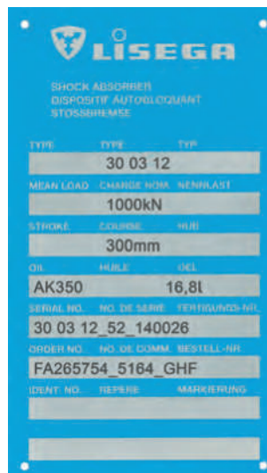
Заводская табличка типа 30
