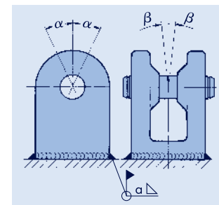
Макс. угловое отклонение, тип 35
