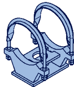
Спец. конструкция типа 49 с ограничителем перемещения
