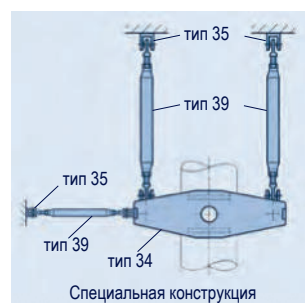
тип 35 тип 39 тип 34 Специальная конструкция
