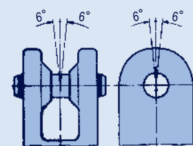
угол нагружения ≤ 6°
