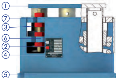
Пружинная опора типа 28 (заблокирована)
