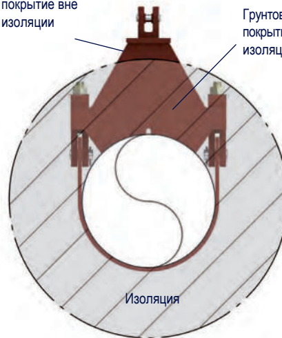
Пример покрытия трубных хомутов с изоляцией для T > 350°C
