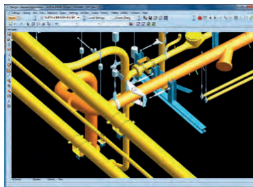
Модель в PDMS™ после импорта данных из LICAD®
