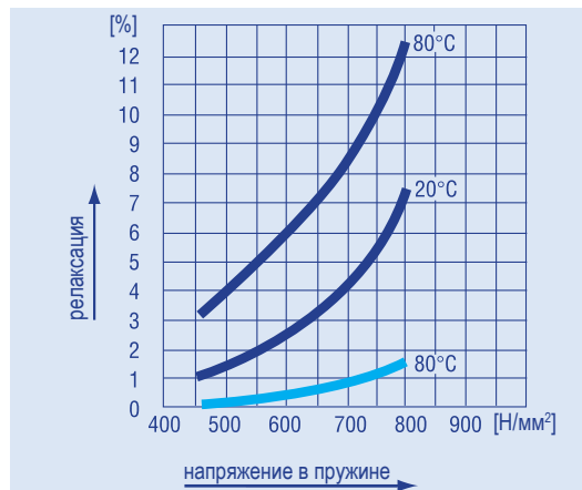
Релаксационные свойства спиральных пружин
