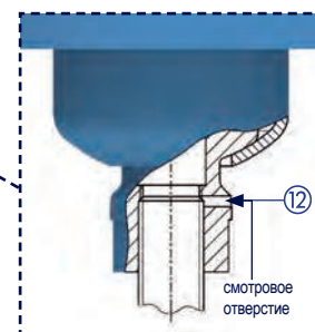
Мин. глубина ввинчивания соединительного стержня в воспринимающую нагрузку трубу
