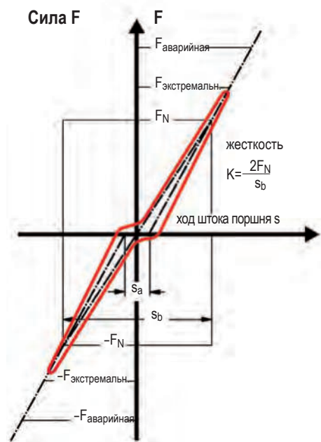
Диаграмма сила - перемещение
