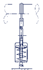
Шарнирная пружинная опора типа 20
