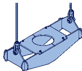
Вертикальный трубный хомут типа 46 с соединениями
