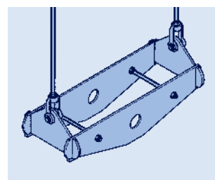
Вертикальный трубный хомут типа 48 с соединительными компонентами
