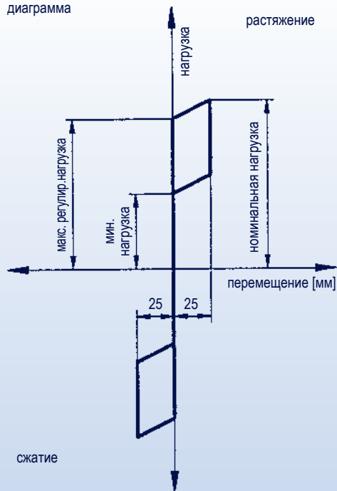
функциональная диаграмма
