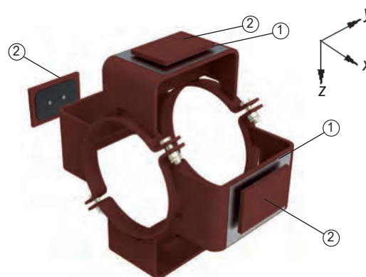
Хомутовая опора типа 49 ... G4-SP, ограничивающая перемещения по осям X-Z с направляющими по оси Y, со скользящими подложками
