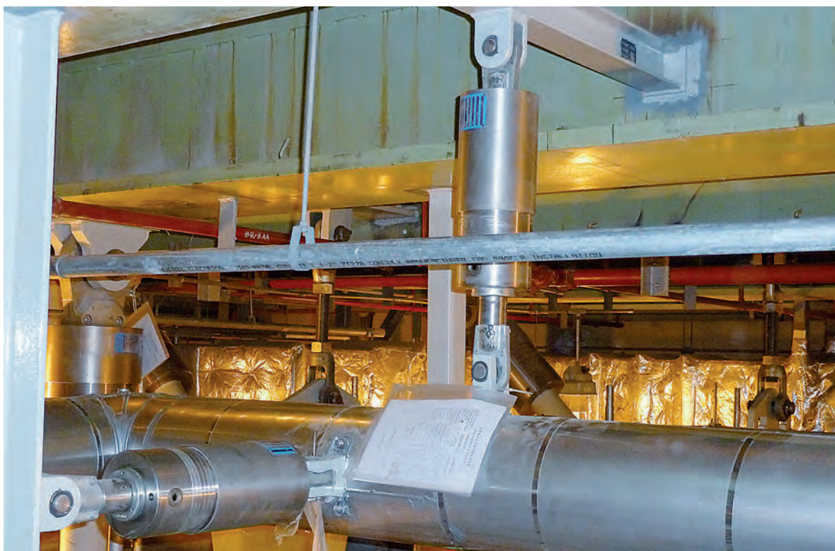
Трубопровод защищен ударными стопорами типа 30, присоединенными к хомутам типа 36
