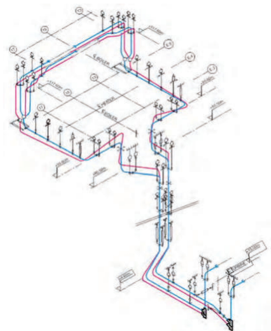
Холодное/горячее положение трубопровода
