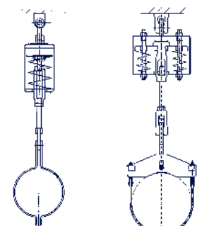
Пруж.подвеска тип 21
