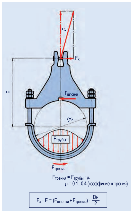
Распределение силы в динамическом хомуте с фиксирующими шпонками
