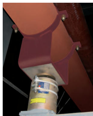
Пластина из нержавеющей стали на основании хомутовой опоры типа 49, теплоустойчивая скользящая подложка и пружинная опора типа 29
