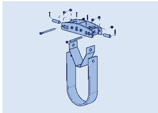
Монтаж типа 44 для температуры выше 600°C
