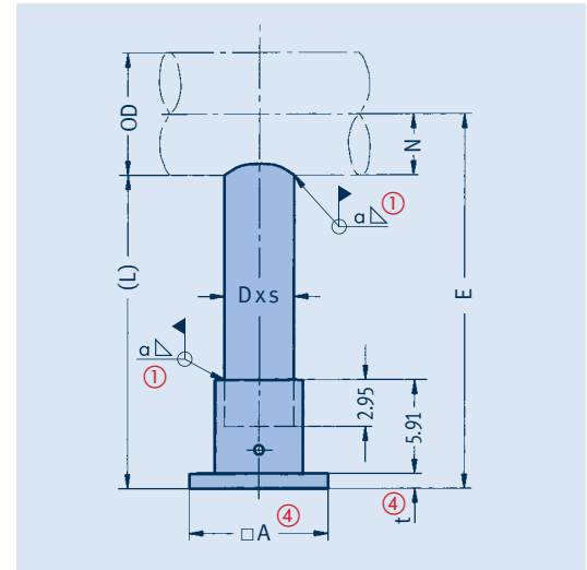
Type 58 .. 21 Type 58 .. 22
