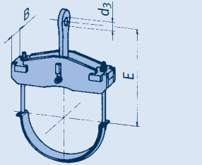
① type 46
