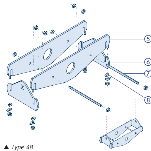
▲ Type 48
