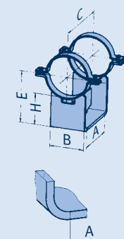
type 49
