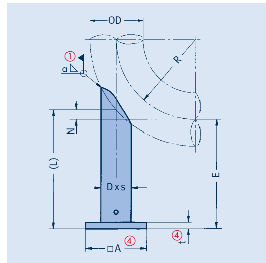
Type 58 .. 15 Type 58 .. 16
