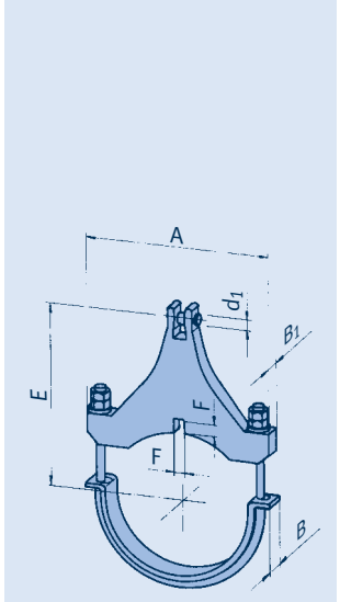
type 36 .. 1/2
