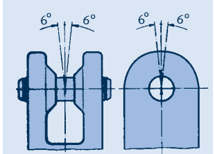
load angle ≤ 6°
