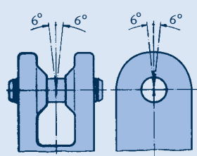
load angle ≤ 6°
