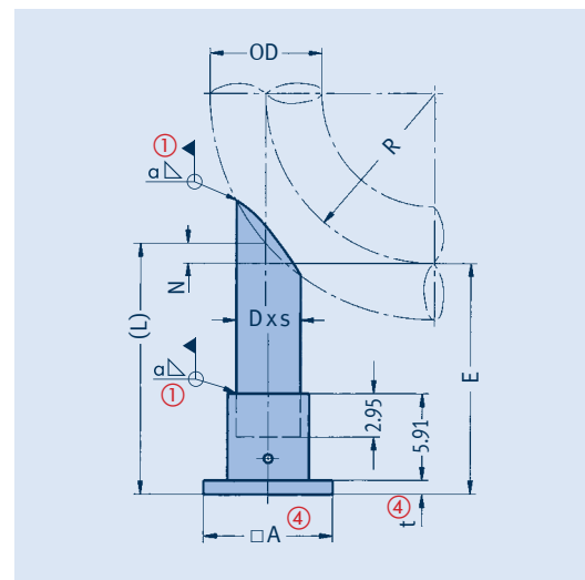
Type 58 .. 25 Type 58 .. 26
