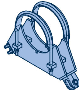
Sonderkonstruktion Typ 38
