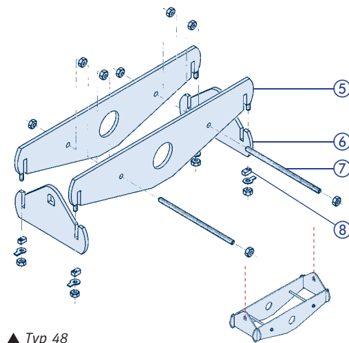
▲ Typ 48
