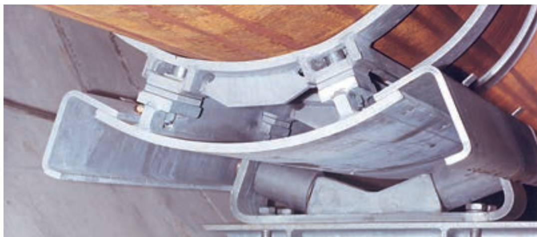
Sonder-Rohrsattel Typ 54 mit Doppelzylinderrollenlager Typ 53 und Abhebesicherungen Typ 55
