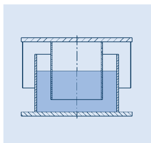
Aufbau des LISEGA-viskoelastischen Dämpfers
