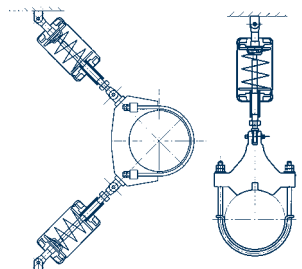
Federstrebe Typ 27 Winkel- anordnung
