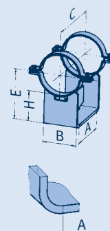
Typ 49
