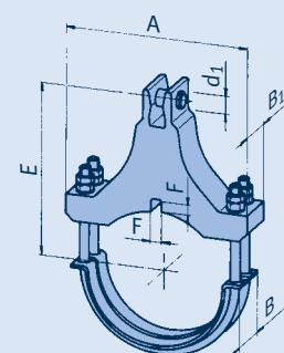
Typ 36 .. .4/5
