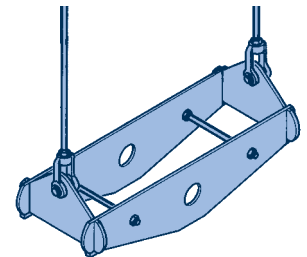
Vertikalschelle Typ 48 mit Anschlussbauteilen
