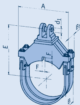
Typ 37 .. .7
