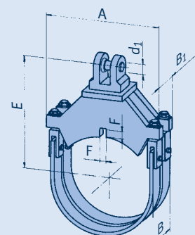
Typ 37 .. .7/8/9
