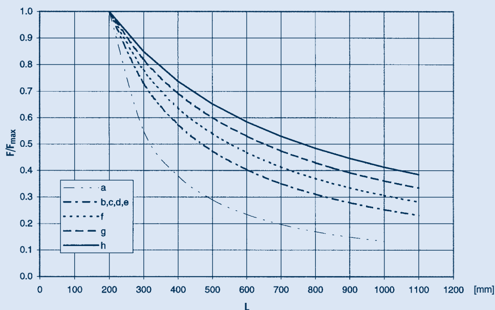
Zulässige Belastung in Abhängigkeit von der Länge der Rohrstütze für Gleitlager bzw. Festpunkt
