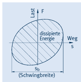
Hysterese eines viskoelastischen Dämpfers
