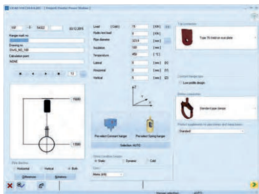
Vue d'ensemble des caractéristiques du support
