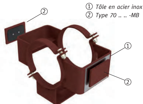
Appuis glissant / patin guide réalisé avec un patin Type 49 ... G3-SP et une plaque de glissement
