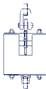
Federhänger Typ 22 mit Gewindebügel Typ 61 montiert
