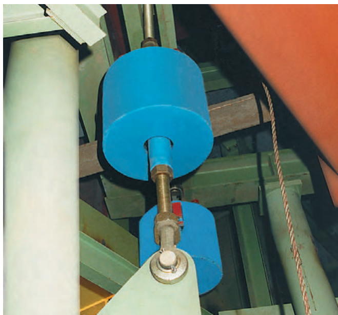
Federhänger Typ 22 mit Gewindebügel Typ 61 montiert
