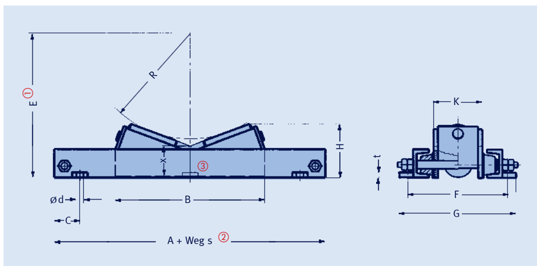
Doppelzylinderrollenlager (seitlich verschiebbar) Typ 53 08 29 bis 53 12 29
