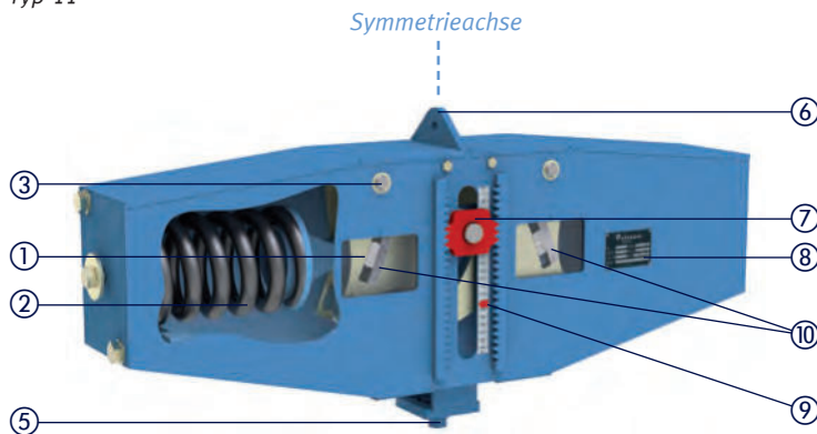
Konstanthänger Typ 18
