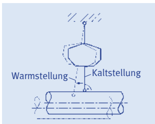
Gestänge senkrecht im Montagezustand
