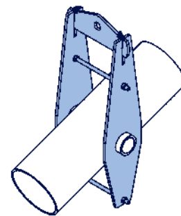
Sonderkonstruktion Typ 48 für eine schräg verlaufende Rohrleitung
