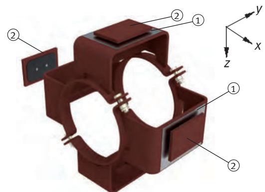
X-Z-Stopp mit Führung in Y-Richtung durch Rohrlager Typ 49 ... G4-SP mit Gleitplatten
