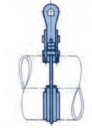
Typ 44 mit Einlageblech
