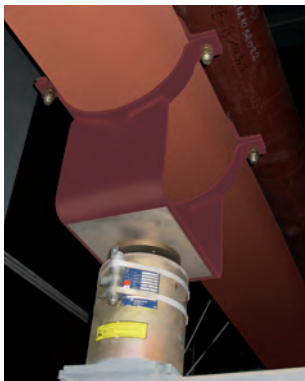
Edelstahl-Gleitblech unter Rohrlager Typ 49, Hochtemperatur-Gleitplatte und Federstütze Typ 29
