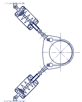
Federstrebe Typ 27 Winkelanordnung
