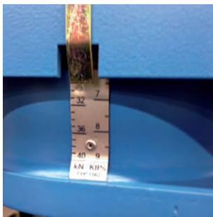
Lastskala mit Anzeiger
