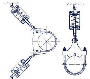
Federstrebe Typ 27 Winkel- anordnung
