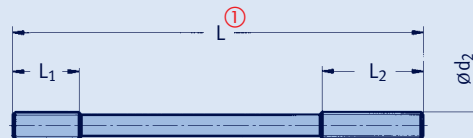
Zugstange Typ 66
