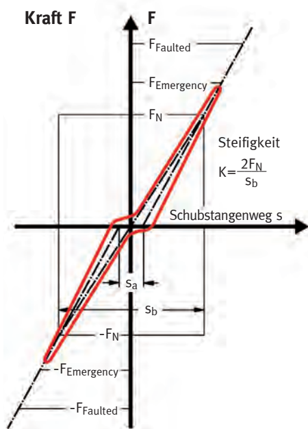
Kraft-Weg Diagramm
