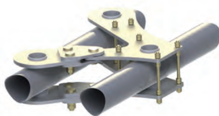
LISEGA-Dreigelenk (Sonderkonstruktion)
