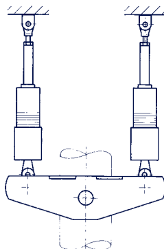
Dynamische Rohrschelle Typ 34 mit Stoßbremsen und Verdrehungen
