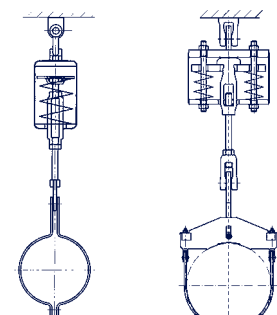
Federhänger Typ 21
