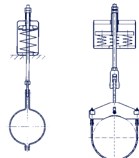
Federhänger Typ 25
