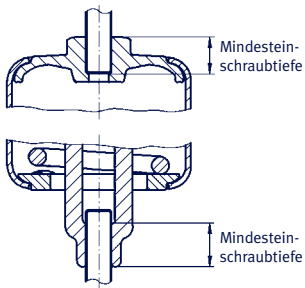
Mindesteinschraubtiefe der Gewindestangen am Beispiel Typ 21
