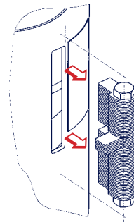
Die Blockierung wird aus dem Gehäuse entfernt
