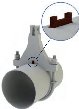
Typ 36 mit Verdreh-sicherung Typ 3L
