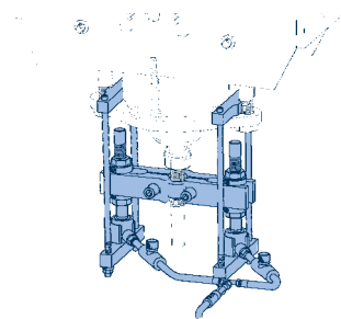
Montagevorrichtung, eingesetzt zur Entlastung der Blockierung
