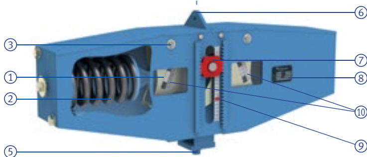
Konstanthänger Typ 18
