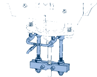
Montagevorrichtung, eingesetzt zur Entlastung der Verstell-schrauben
