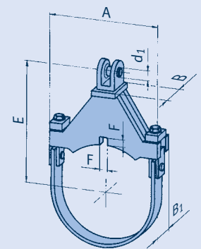
Typ 37 .. .1/2/3/4/5/6
