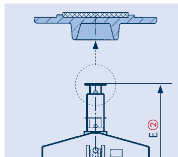
Laststeller mit integrierter Gleitplatte
