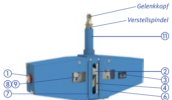
Konstantgelenkstütze Typ 19
