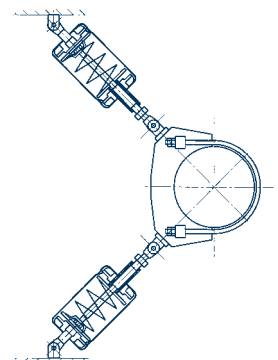
Federstrebe Typ 27 Winkelanordnung
