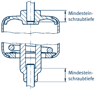
Mindesteinschraubtiefe der Gewindestangen am Beispiel Typ 21
