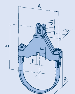
Typ 37 .. .1/2/3/4/5/6
