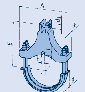
Typ 36 .. .4/5
