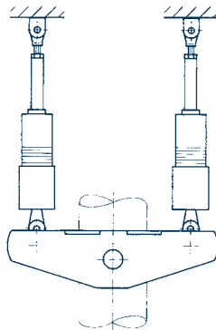
Dynamische Axialschelle mit Stoßbremsen
