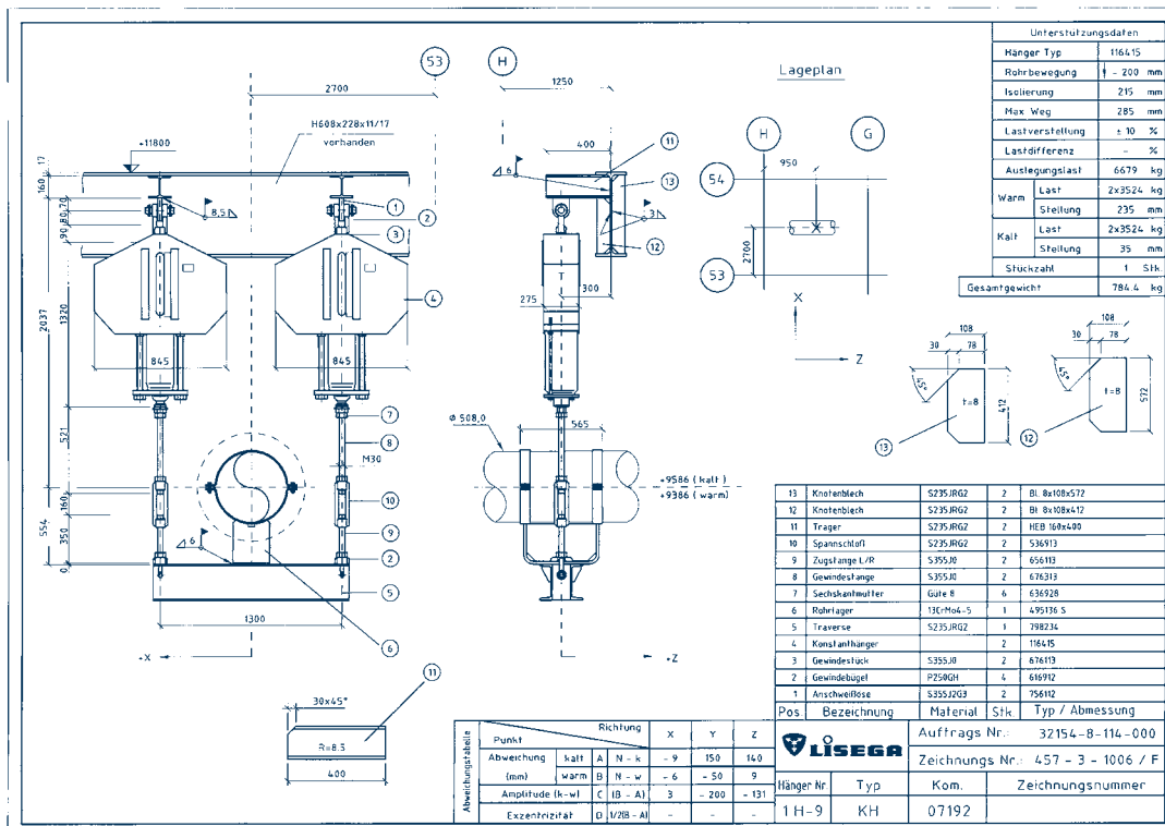
AutoCAD®-Zeichnung, erstellt auf der Grundlage einer LICAD®-Konstruktion
