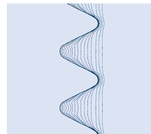
Faserverlauf gerollter Gewinde
