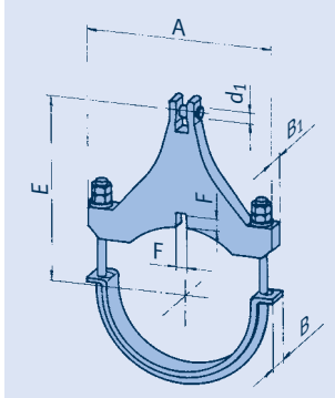
Typ 36 .. .1
