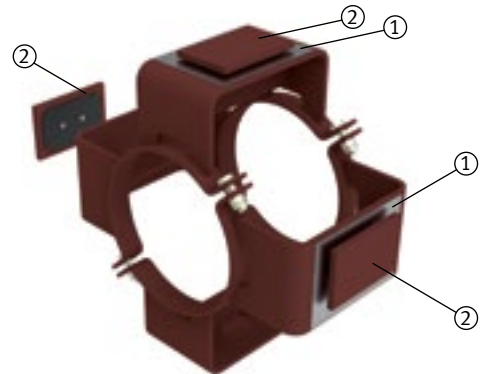
X-Z-Stopp mit Führung in Y-Richtung durch Rohrlager Typ 49 .. .. -G4-SP mit Gleitplatten
