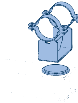
Typ 43 mit Einlageblech
