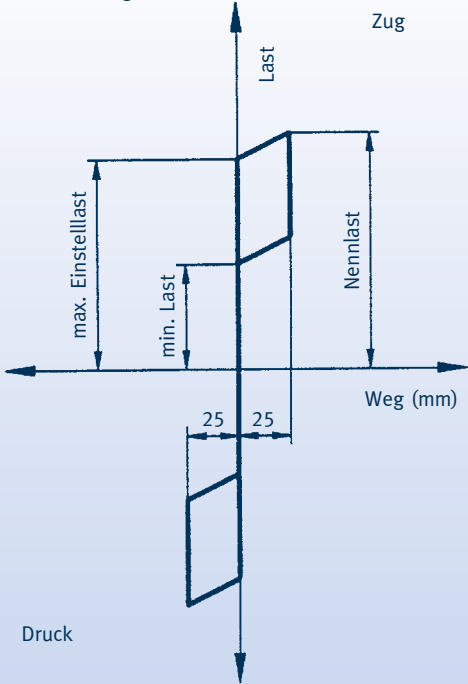
Funktionsdiagramm
