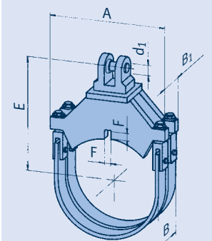
Typ 37 .. .8/9
