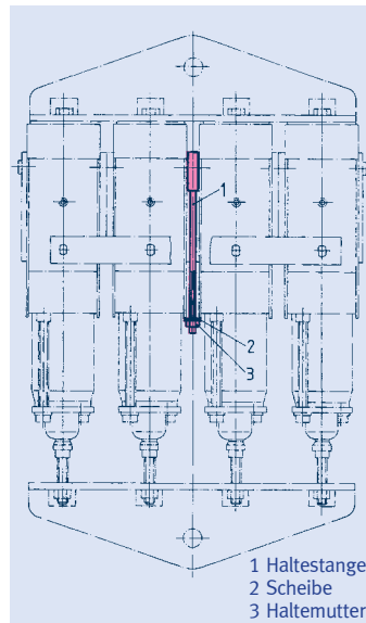
Transportsicherung Typ 12 82 .. – 14 96 ..
