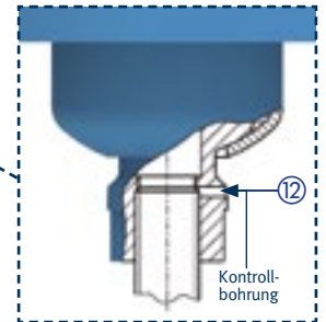
Mindest-Einschraubtiefe des Anschlussgestänges im Laströhre
