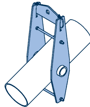
Sonderkonstruktion Typ 48 für eine schräg verlaufende Rohrleitung
