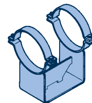
Bauart 2: Rohrlager für mittlere und hohe Temperaturen Typ 49 .. .3, .. .4, .. .5
