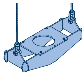
Vertikalschelle Typ 46 mit Anschlussbauteilen
