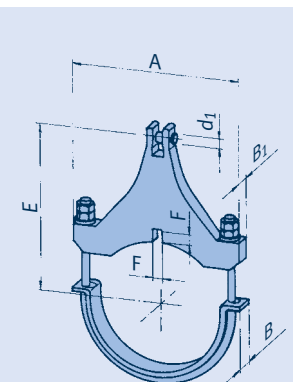
Typ 36 .. .1/2/3
