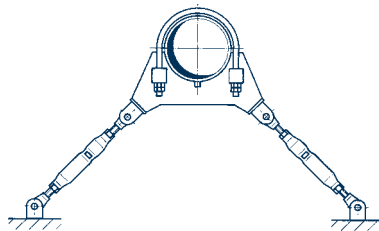
Sonderschelle für die Winkelanordnung
