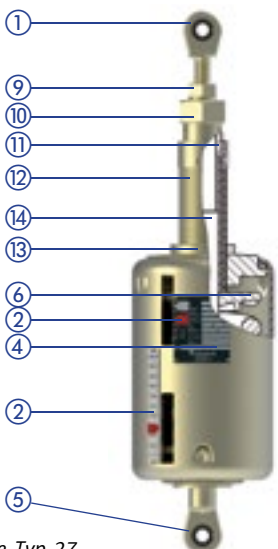
Federstrebe Typ 27
