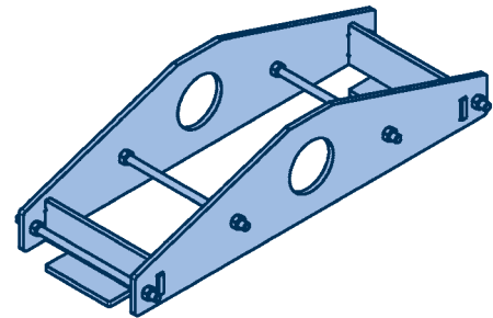
Sonderkonstruktion Typ 48 (aufgesetzt)
