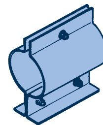
Bauart 1: Rohrlager für niedrige Temperaturen Typ 49 .. .1, 49 .. .2 bis NW150
